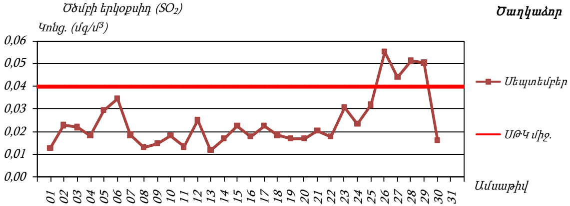
Ծաղկաձոր քաղաքի մթնոլորտային օդում ծծմբի երկօքսիդի կոնցենտրացիաների փոփոխությունները.
